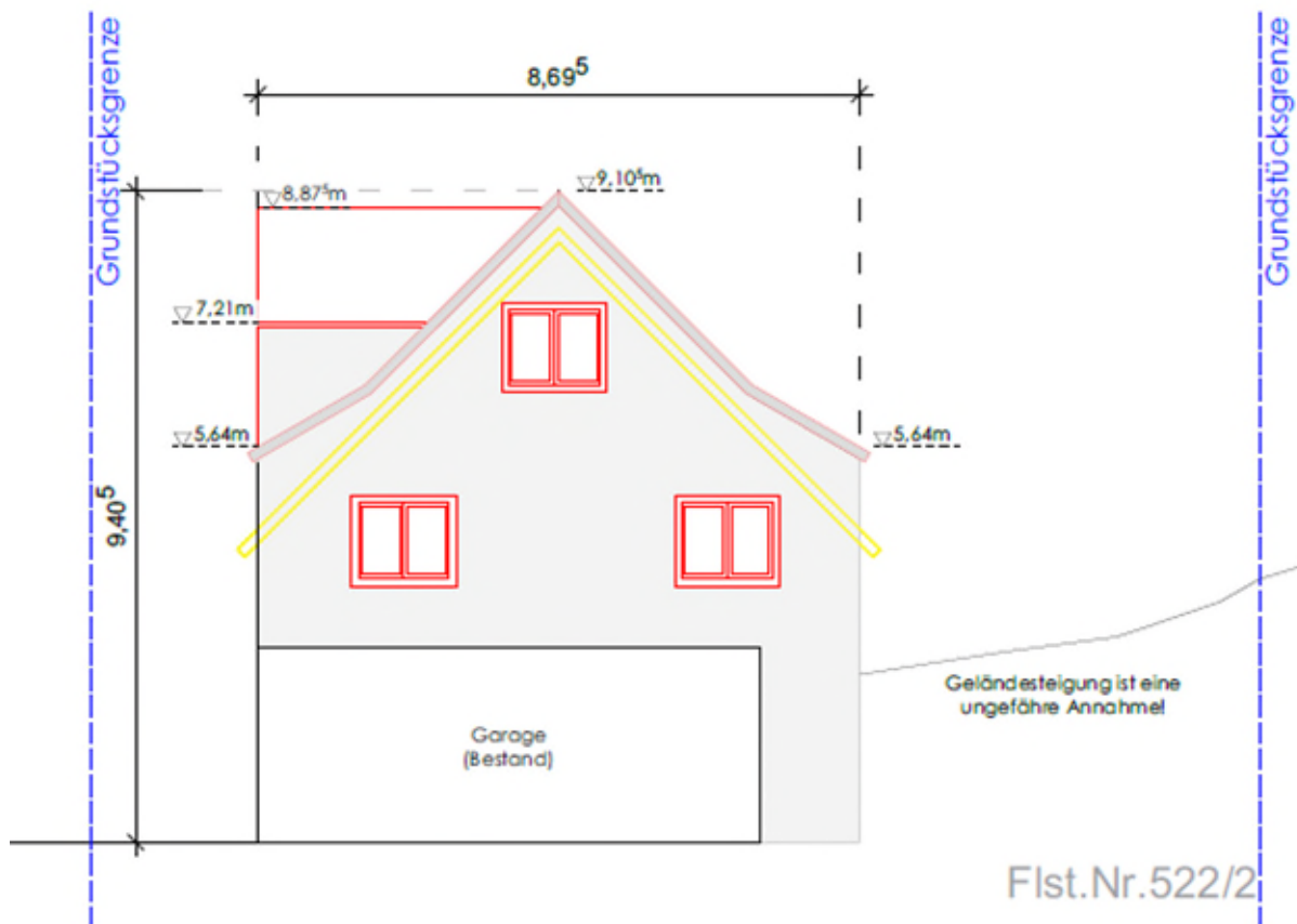
Ansicht Ost
