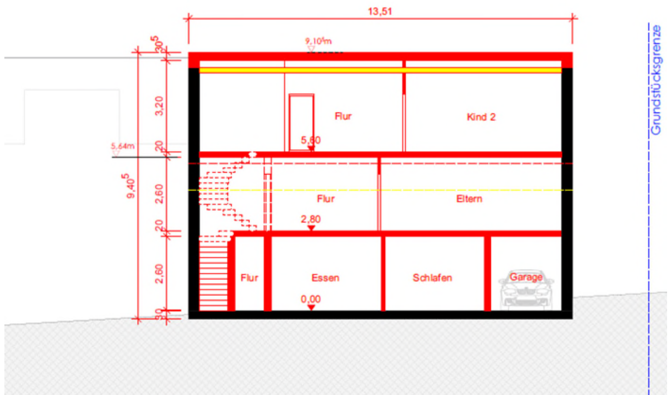
Schnitt
