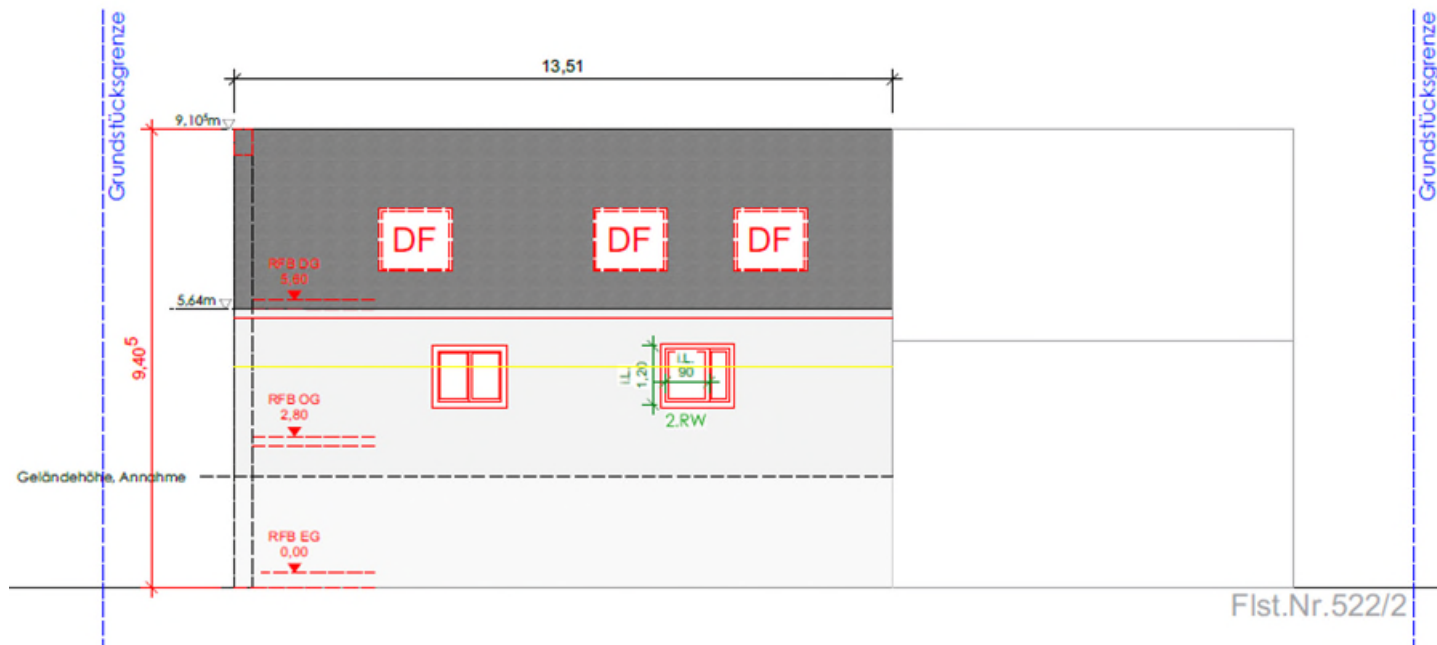
Ansicht Nord
