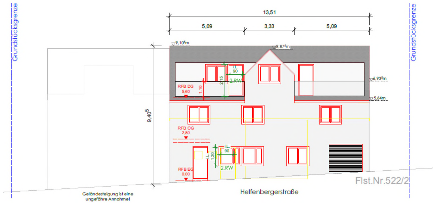
Ansicht Süd
